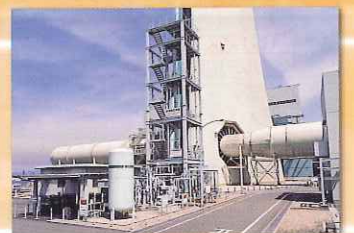
関西電力(株)CO 2 分離回収パイロットプラント
